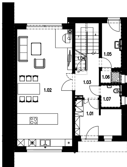
1. NP
