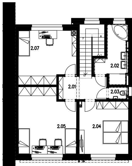
2. NP
